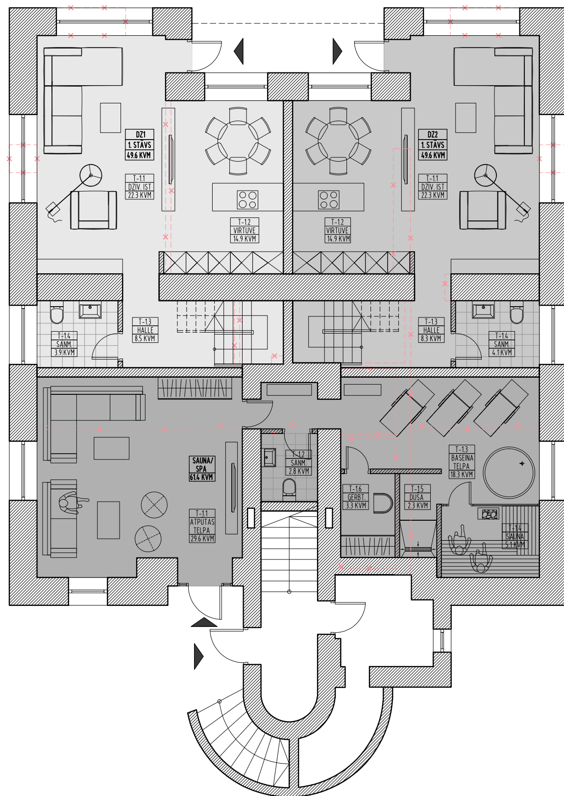
1. STĀVA PLĀNS
