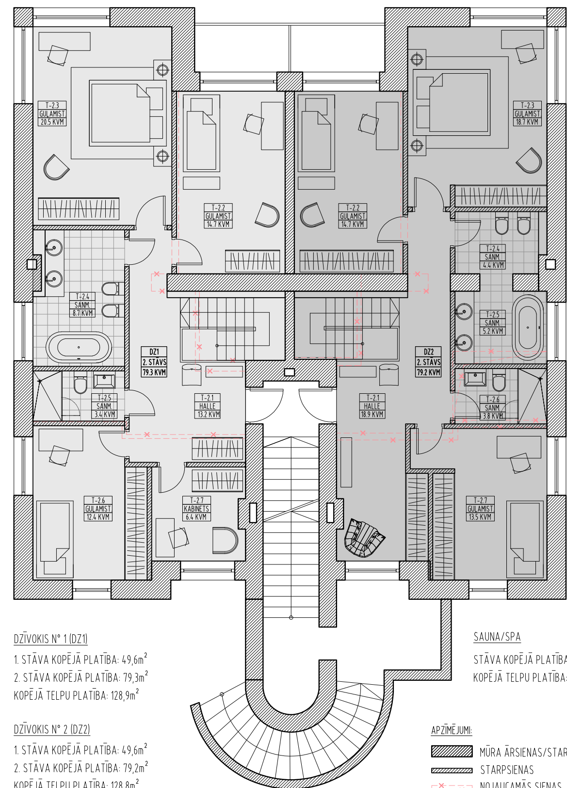
2. STĀVA PLĀNS
