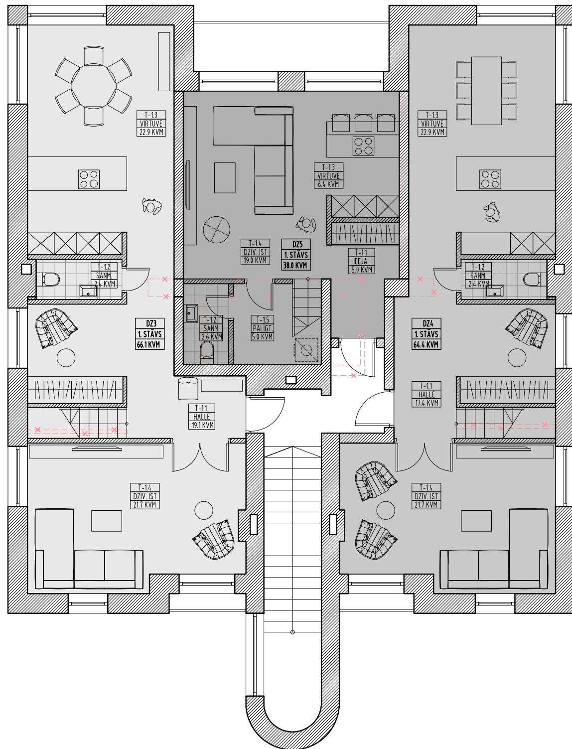
3. STĀVA PLĀNS
